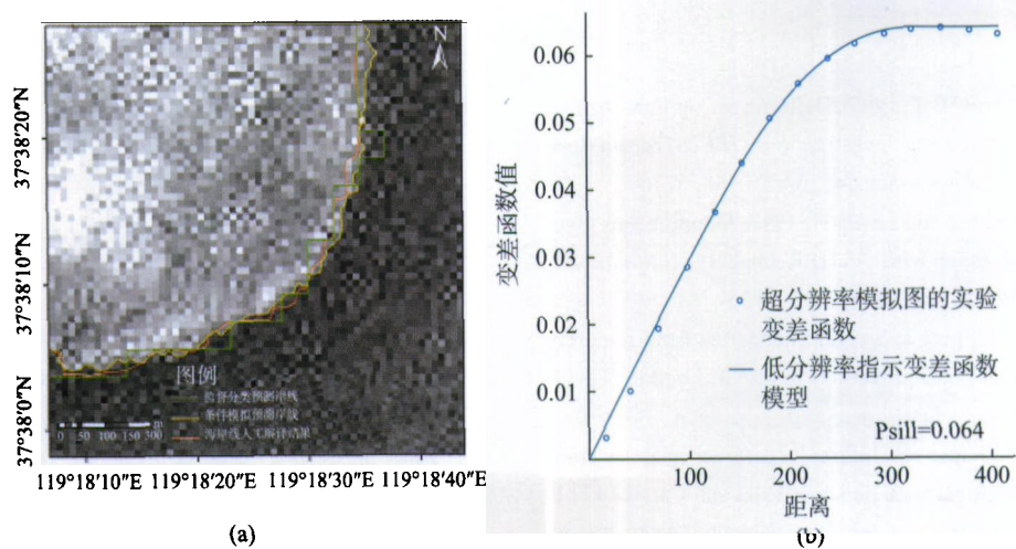
图 7 (a) 黄河河口段淤泥质海岸应用于原始图像的监督分类预测岸线与应用于 SIcS 图像的条件模拟预测岸线之间的比较; (b) 由模拟概率均值计算得到的变差函数
